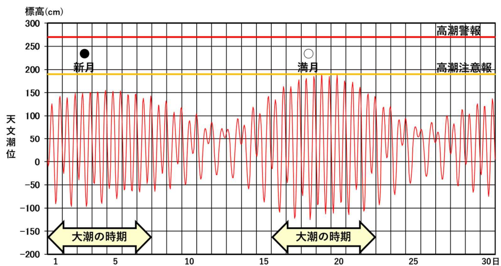
図3 苓北における2024年9月（1時間ごとの）の天文潮位
